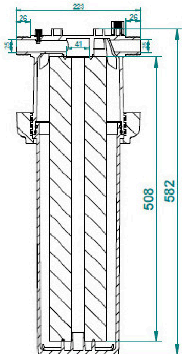
SECTION A-A
