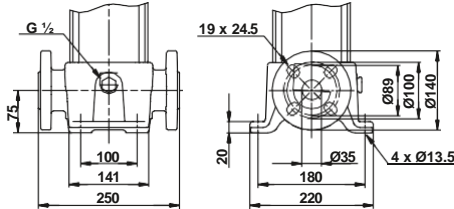
FGJ (DIN-ANSI-JIS) PN 25 / DN 32
