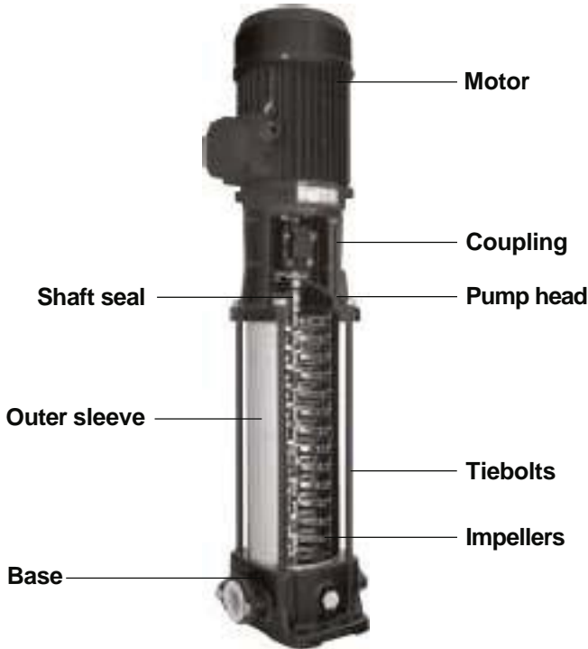
Fig. 2 LCR pump
